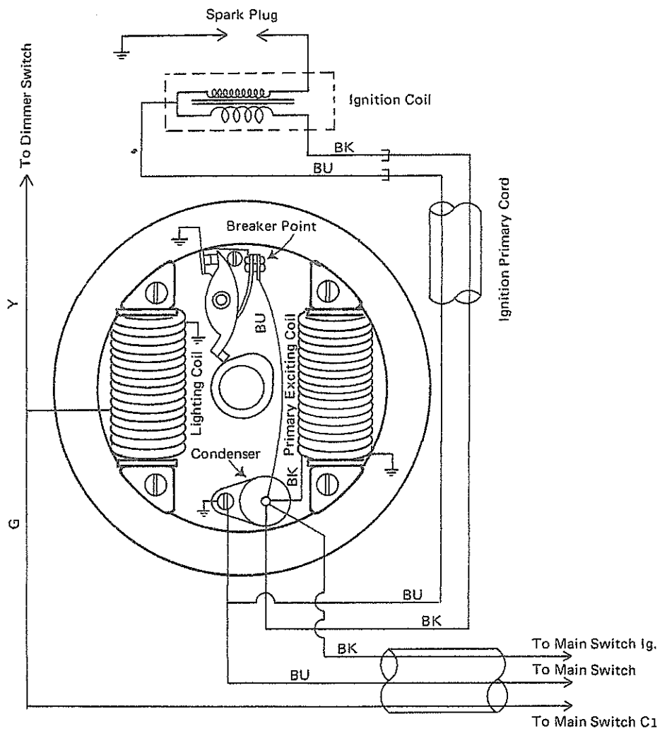
Fig. 6A Magneto/Alternator Wiring Diagram
